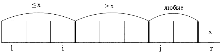
Рис. 5.4. К алгоритму быстрой сортировки
