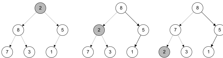
Рис. 9.20. Восстановление свойства кучи
