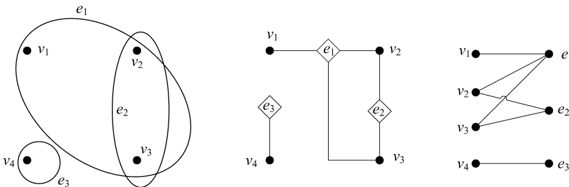
Рис. 7.29. Диаграммы гиперграфов
