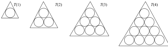
Рис. 1.3. Треугольные числа
