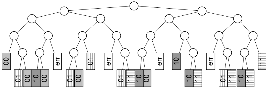
Рис. 6.3. Дерево решений
