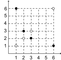
Рис. 1.9. К примеру 1.4.8
