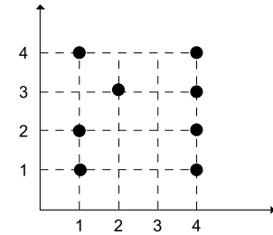
Рис. 1.8. К примеру 1.4.6
