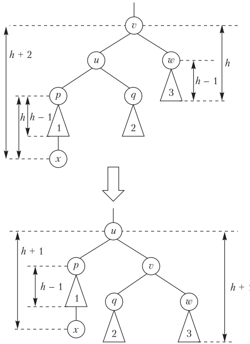
Рис. 9.17. Простое вращение
