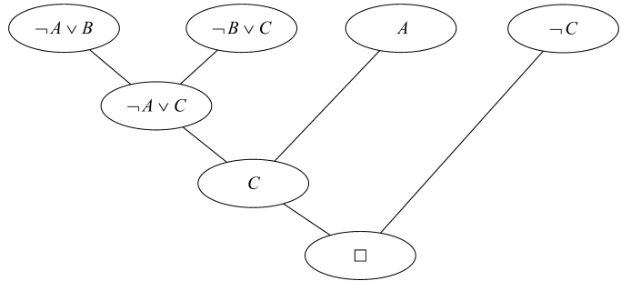
Рис. 4.2. Дерево вывода 1
