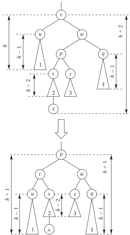
Рис. 9.18. Двойное вращение
