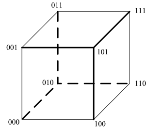
Рис. 6.1. Гиперкуб
