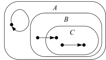
Рис. 1.1. К доказательству теоремы 1.2.3
