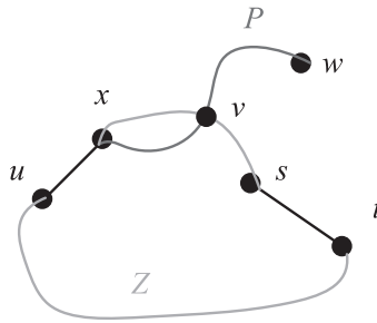
Рис. 8.5. К доказательству пункта [4 \Rightarrow 5] теоремы о блоках
