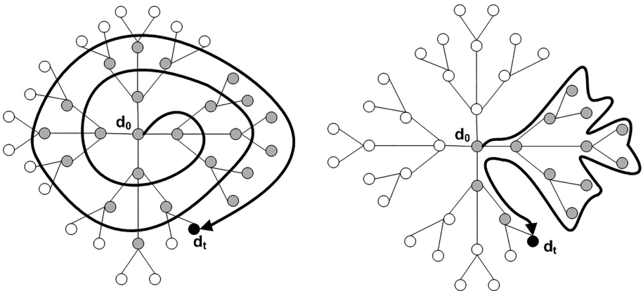
Рис. 7.22. Обходы в ширину и глубину
