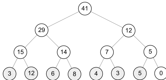
Рис. 9.21. Дерево отрезков
