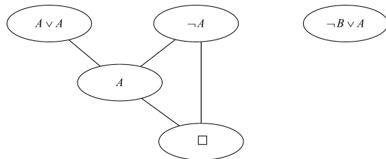
Рис. 4.3. Дерево вывода 2
