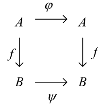
Рис. 2.2. Коммутативная диаграмма
