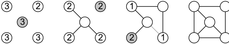
Рис. 7.11. Откладывание вершин
