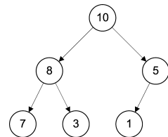
Рис. 9.19. Двоичная куча
