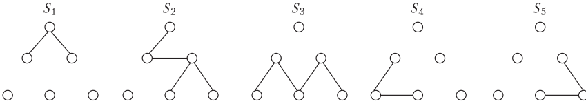
Рис. 10.5. Фундаментальные разрезы
