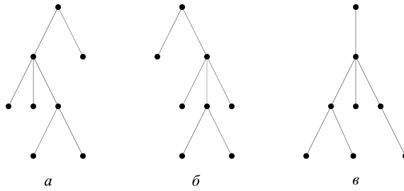
Рис. 9.9. Диаграммы деревьев
