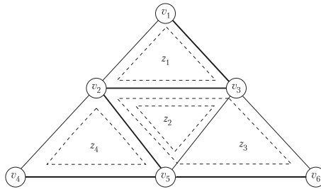
Рис. 10.4. Фундаментальные циклы
